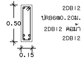
แบบขยายคาน 1:25
