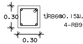
ดอมม่อ 1:25
