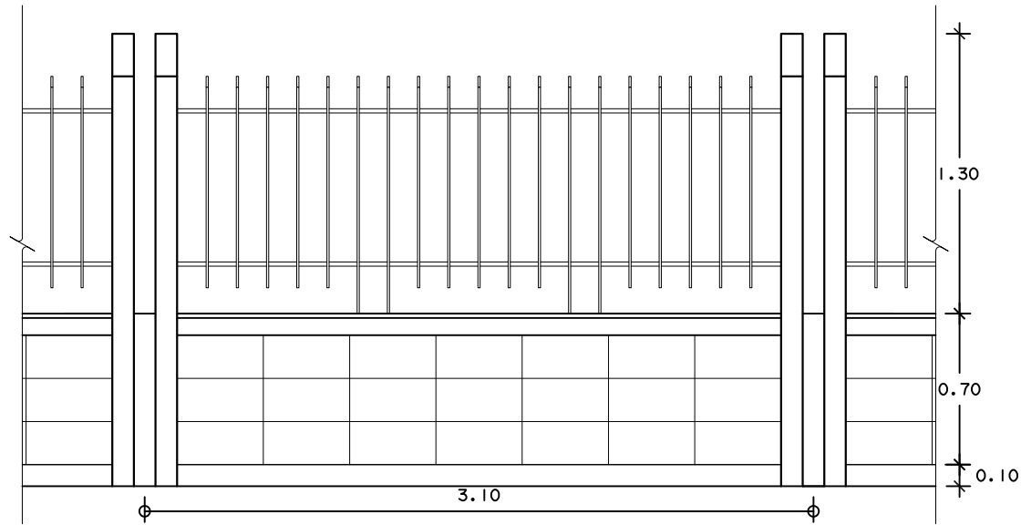
รูปด้าน(แบบโปร่ง) 1:25
