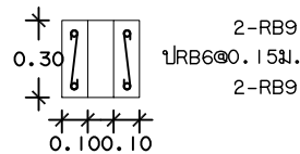
เสาร้ว 1:25
