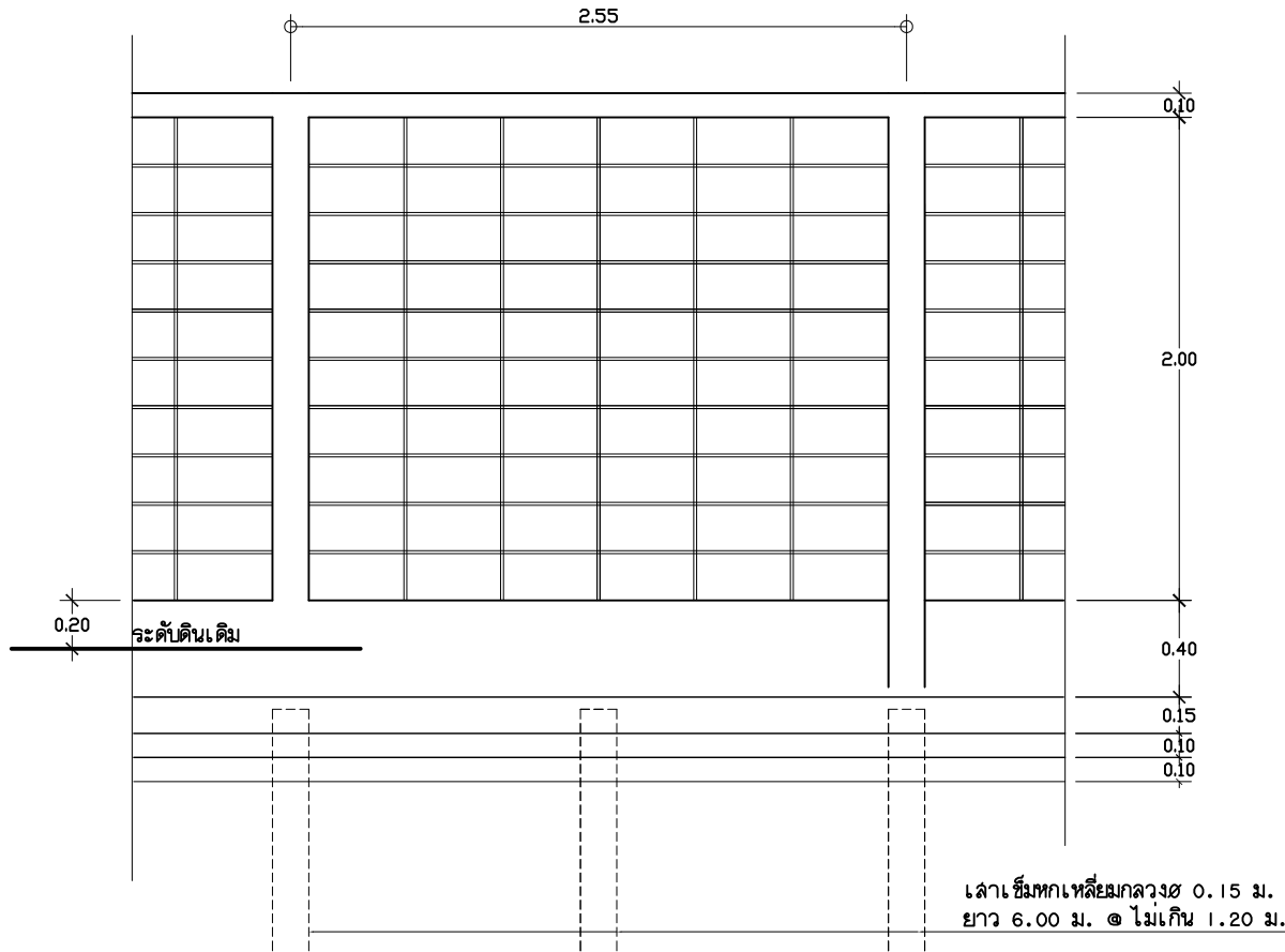
รูปด้าน มาตรการส่วน 1 : 25
