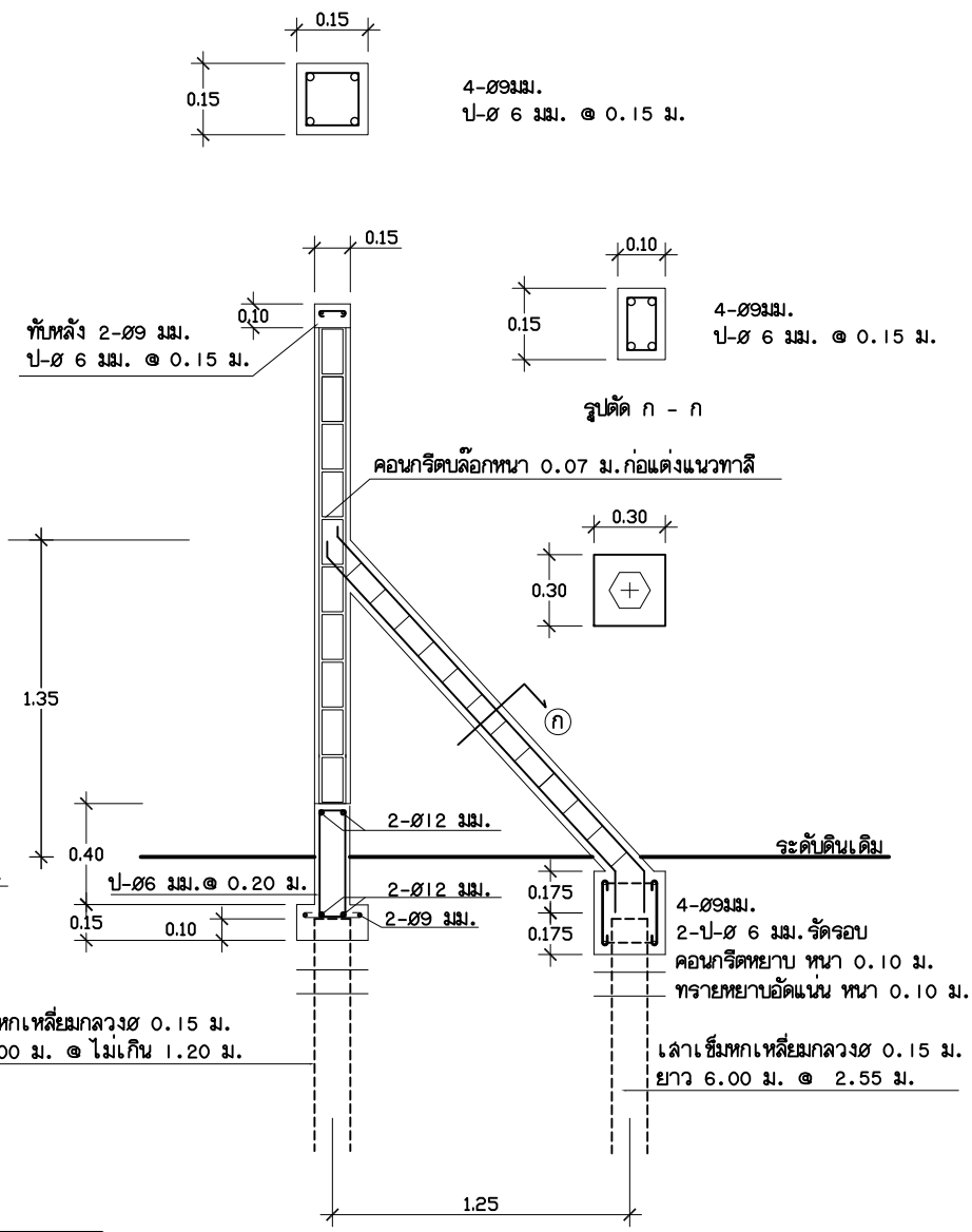
รูปตัด มาตรการส่วน 1 : 25
