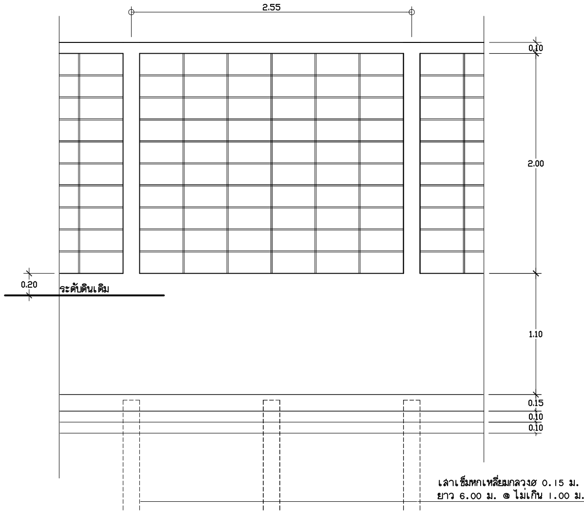
รูปด้าน มาตรการส่วน 1 : 25
