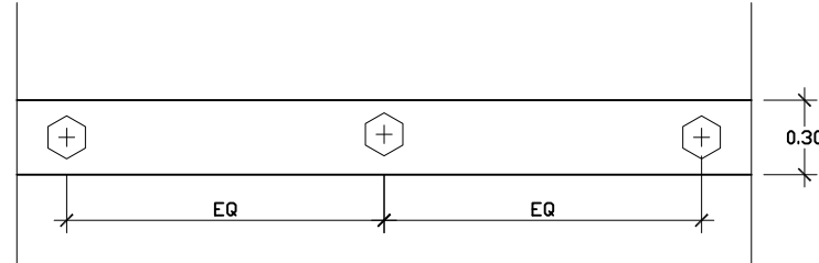
แบบแปลน มาตรการส่วน 1 : 25
